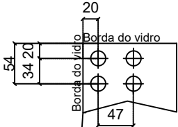
Furação instalação
