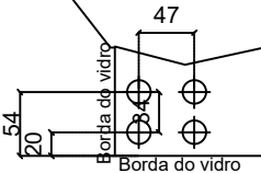
Furação instalação
