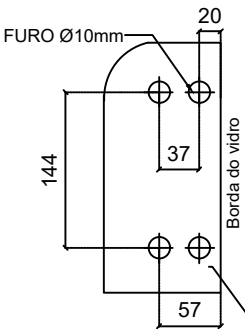
Furação instalação
