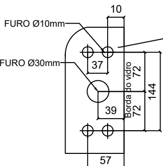
Furação instalação
