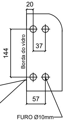
Furação instalação
